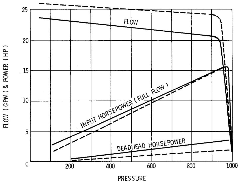
TV-40 @ 1200 rpm
