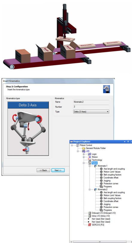
Intégration de la fonction robot avec IndraMotion for packaging Photo : Bosch Rexroth AG
