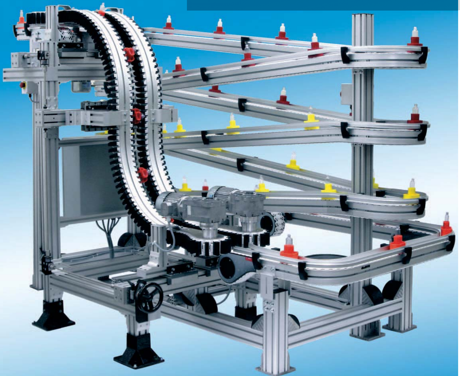
Systeme de transport à chaîne VarioFlow S
