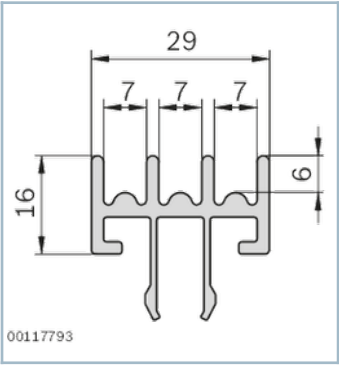
Sliding door profile, bottom
