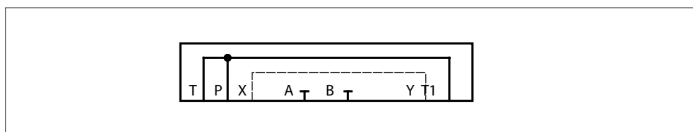
Abb. 2: Spülplatte, Darstellung der inneren Verbindungen
