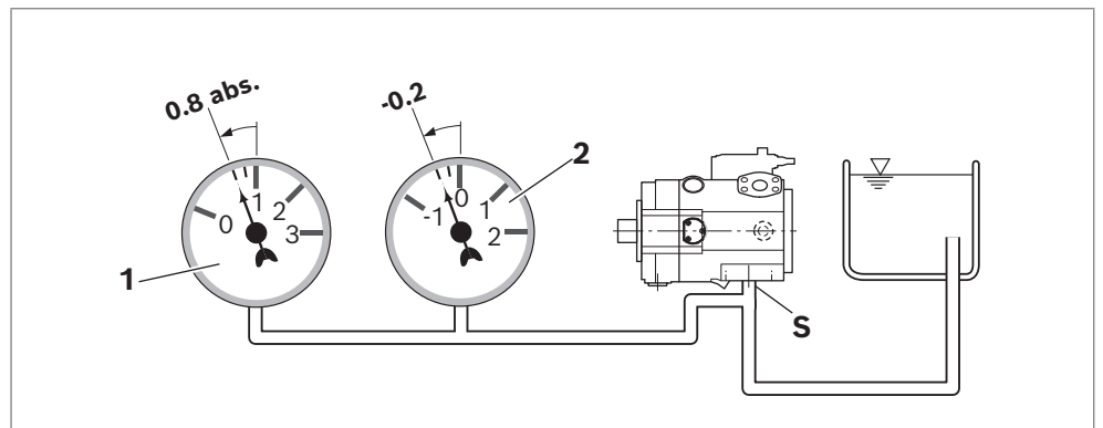
Abb. 7: Saugdruck
