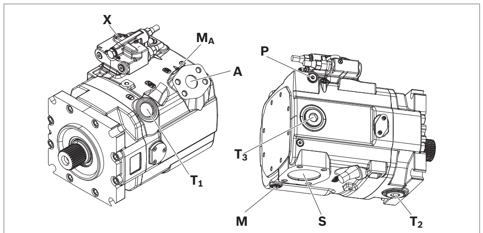
Abb. 11: Anschlussübersicht A15VSO mit LRDRS0-Verstellung, Drehrichtung rechts
