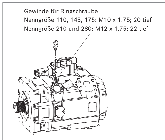
Abb. 5: Befestigung der Ringschrauben im Gehäuse oben
