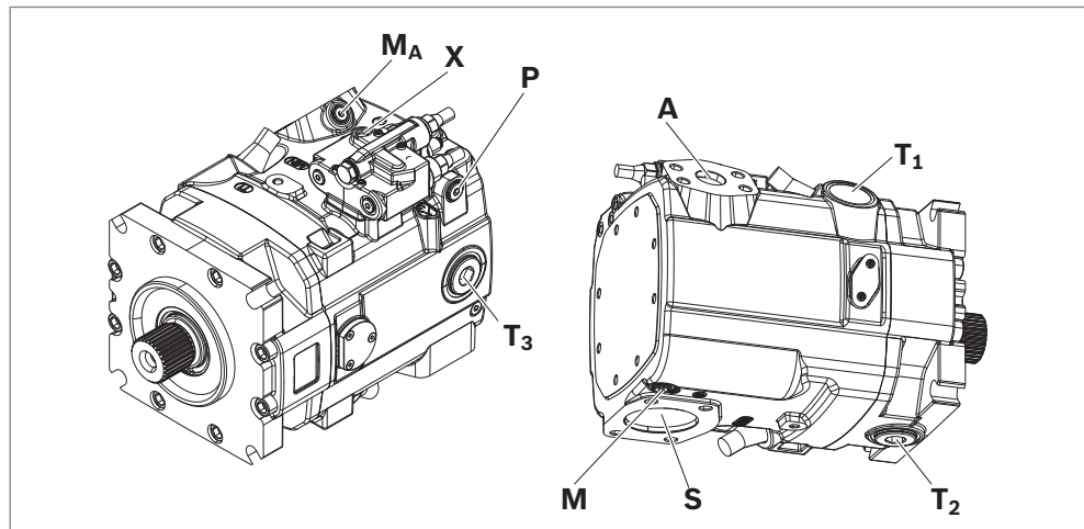
Abb. 12: Anschlussübersicht A15VSO mit LRDRS0-Verstellung, Drehrichtung links
