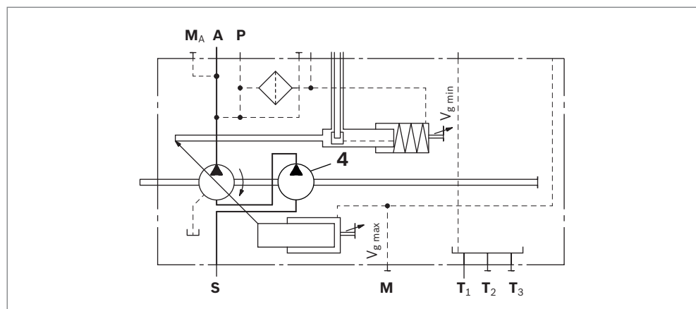
Abb. 3: Schaltplan A15VLO mit Ladepumpe
