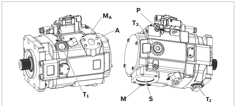
Abb. 10: Anschlussübersicht A15VLO mit E2DR-Regler, Drehrichtung rechts
