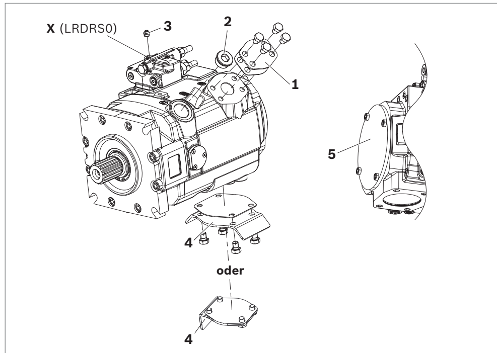
Abb. 9: Transportschutz entfernen
