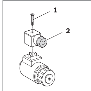
Abb. 13: Hirschmann-Stecker
