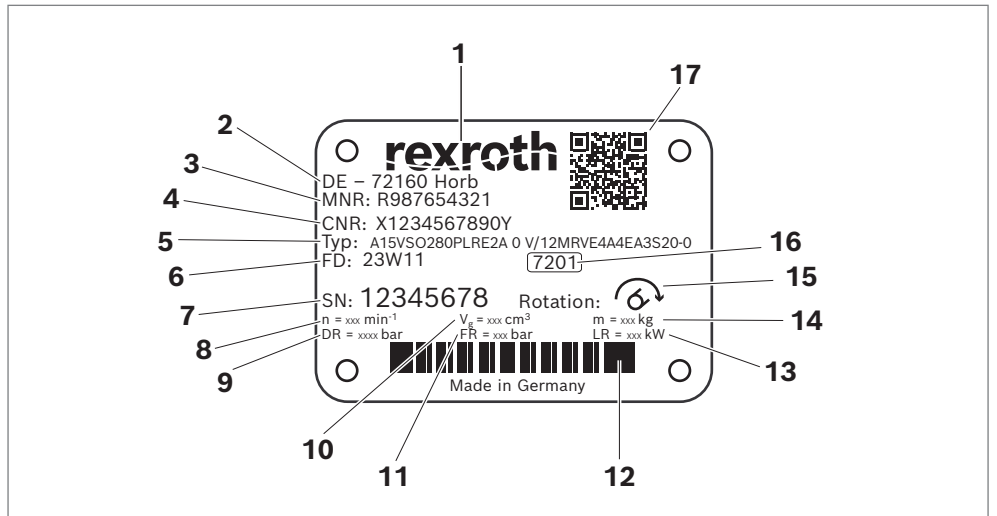
Abb. 4: Typschild A15VSO
