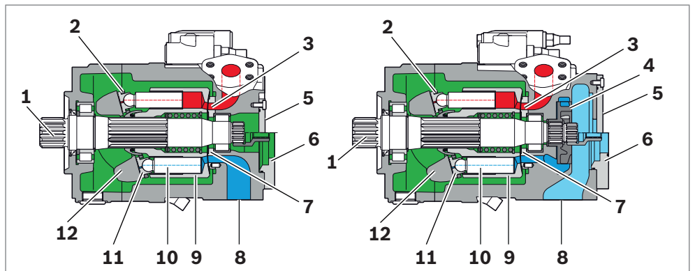
Abb. 2: Linke Darstellung: Aufbau der A15VSO; rechte Darstellung: Aufbau der A15VLO
