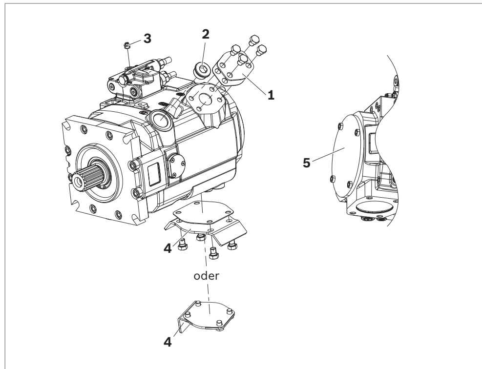
Abb. 1: Axialkolbeneinheit
