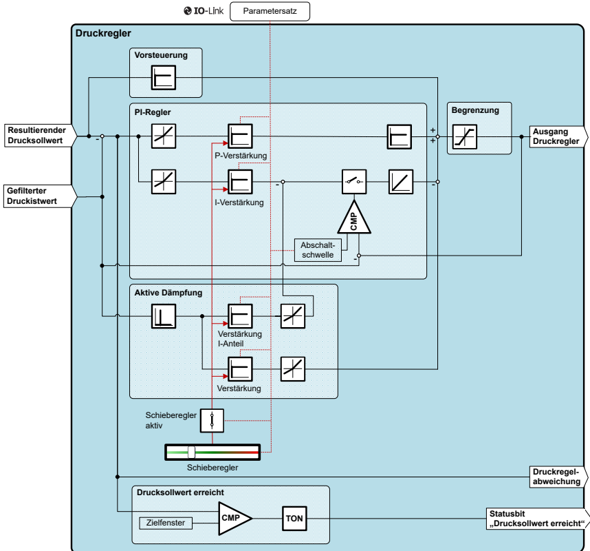
Abb. 50: Druckregelung
