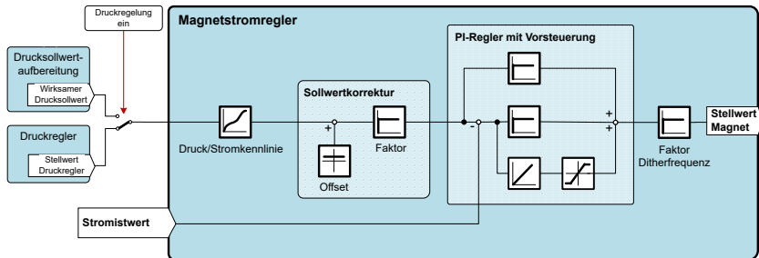
Abb. 52: Magnetstromregler
