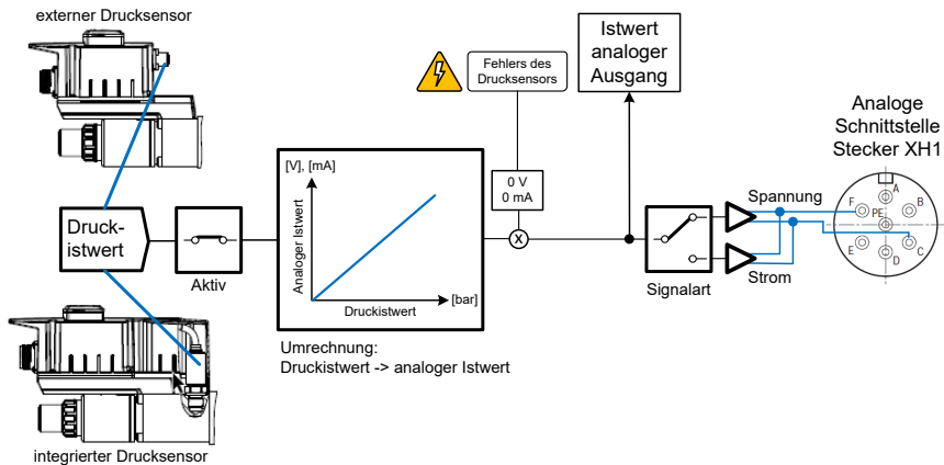
Abb. 16: Druckistwert1
