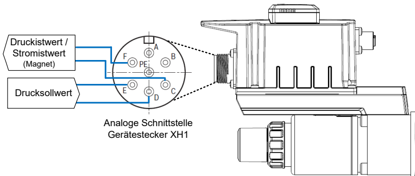
Abb. 7: AnalogeSchnittstelle_Gerätesteckerbelegung
