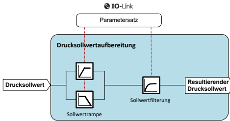
Abb. 47: Drucksollwertaufbereitung1
