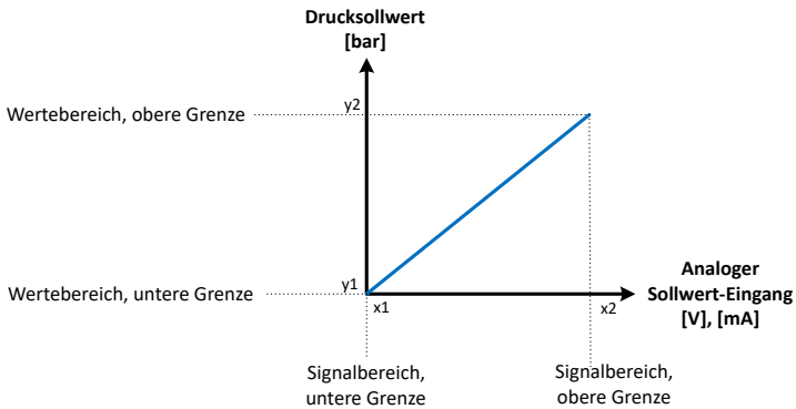
Abb. 9: Drucksollwert3
