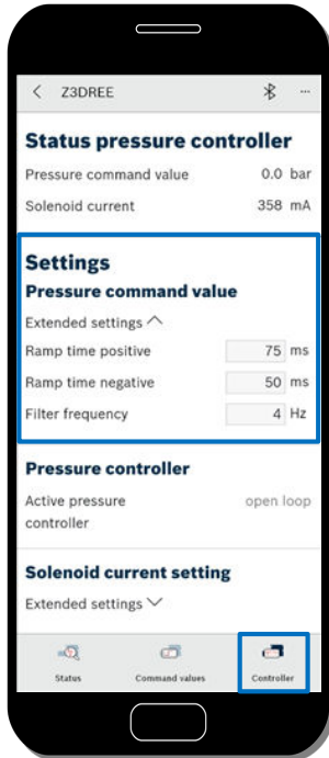
Abb. 48: Drucksollwertaufbereitung2
