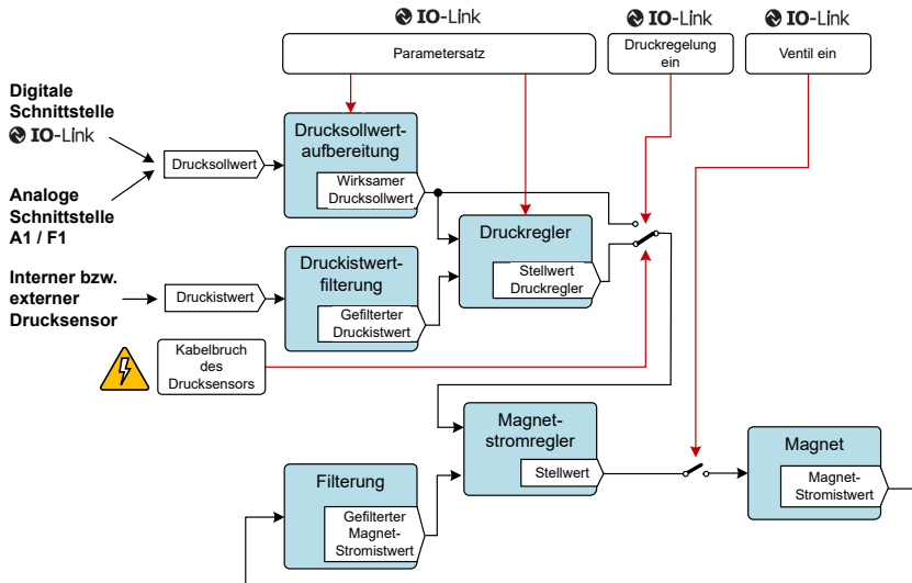
Abb. 45: Reglerstruktur3
