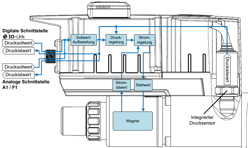
Abb. 3: Übersicht_(Z)3DREA_Drucksensor_integriert
