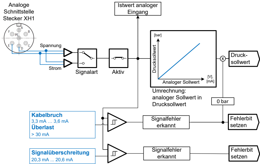
Abb. 8: Drucksollwert1
