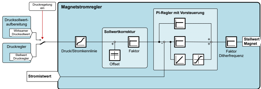
Abb. 43: Magnetstromregler
