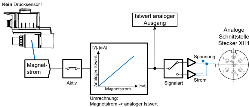
Abb. 24: Stromistwert1
