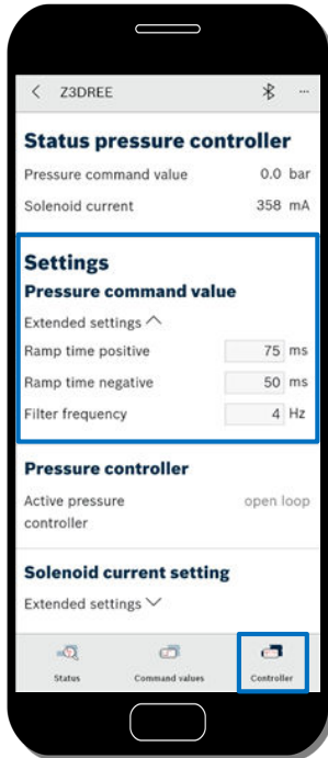
Abb. 42: Drucksollwertaufbereitung2
