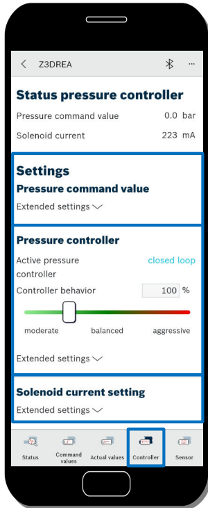
Abb. 46: Reglerstruktur4
