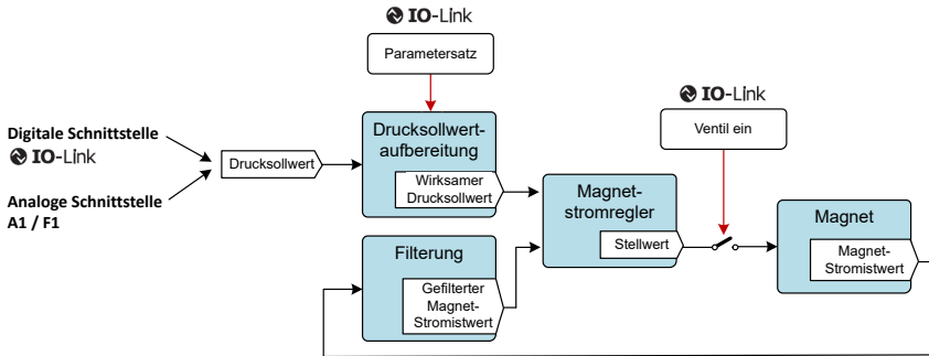
Abb. 39: Reglerstruktur1
