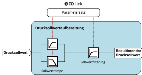
Abb. 41: Drucksollwertaufbereitung1
