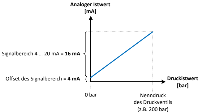
Abb. 21: Druckistwert5
