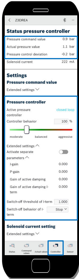
Abb. 51: 29283-FK_Druckregelung2
