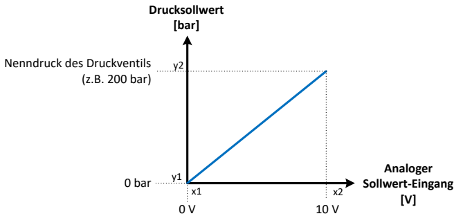
Abb. 11: Drucksollwert4
