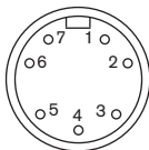
Abb. 2: Servo-Motor: Anschlussbuchse, 7polig (female, Blick auf Servo-Motor)
