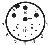
Abb. 1: Servo-Motor: Anschlussbuchse , 14polig (male; Blick auf Servo-Motor)
