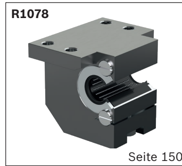
Linear-Set seitlich offen, einstellbar
