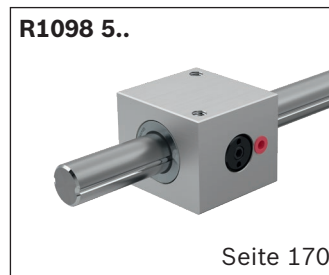
Typ 2: zwei Laufbahnrippen
