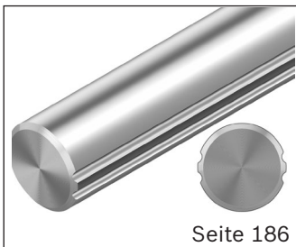
Präzisions-Stahlwelle mit vier Laufbahnrillen
